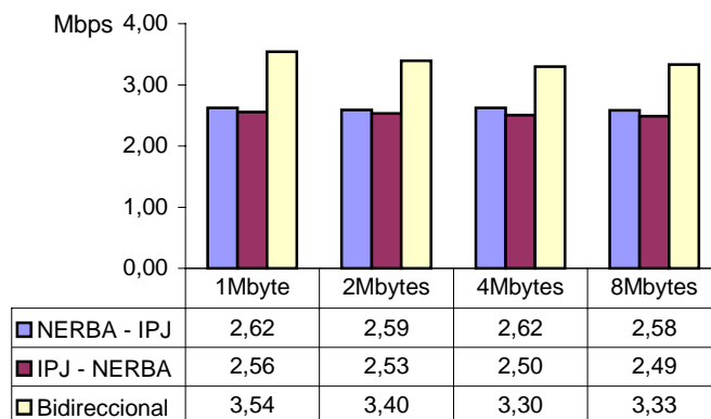
Gráfico 1- Desempenho da ligação NERBA – IPJ
