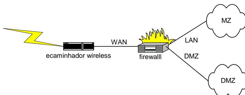
Figura 4 – Topologia local típica.
