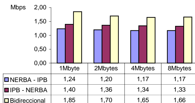
Gráfico 2 – Desempenho da ligação NERBA – IPB
