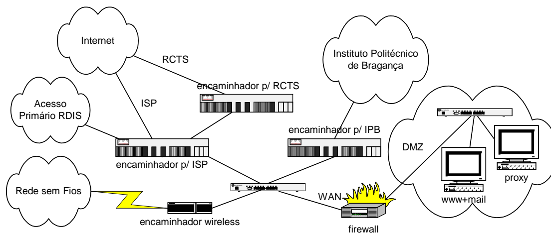
Figura 5 – Topologia no ponto de acesso à Internet (IPB).
