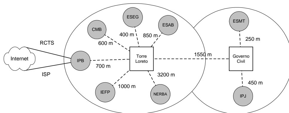
Figura 3 – Topologia à escala metropolitana.
